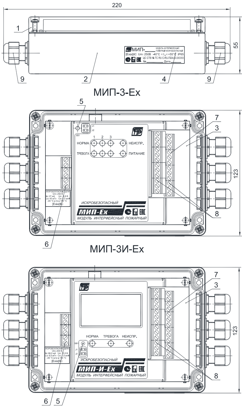
Рис. А1. Внешний вид модулей МИП в настенном исполнении.
